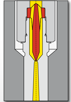
Diverse varianti di boccole di iniezione e boccole avvitata, inclusi modelli allungati da adattare alla forma del pezzo
