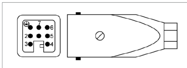
Abbildung 10: Digital Out Signalausgang 8-polig (5)
