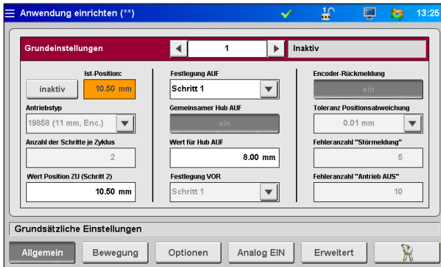
Abbildung 18: Ansicht "Grundeinstellungen"
