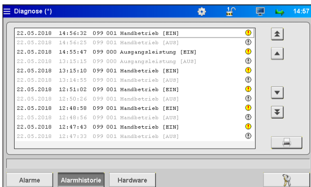
Abbildung 25: Ansicht "Alarmerhistorie"
