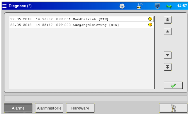
Abbildung 24: Ansicht "Alarmer"
