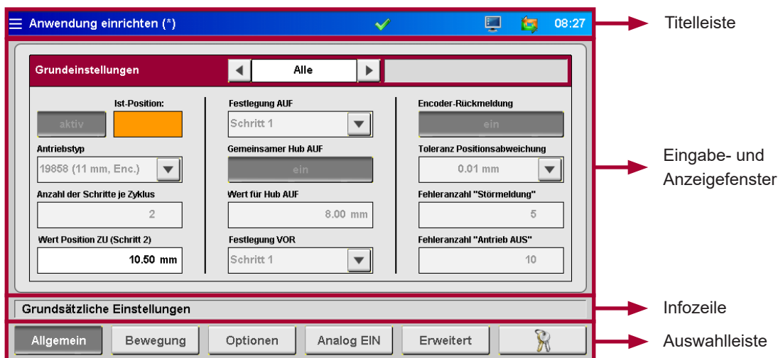
Abbildung 15: Bildschirmaufbau des EDC-PRO Steuergeräts
