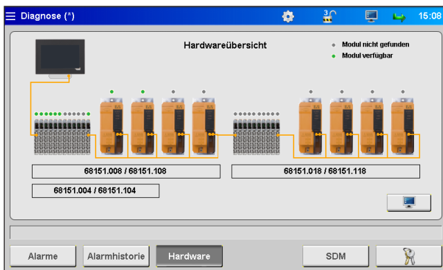
Abbildung 26: Ansicht "Hardwareübersicht"
