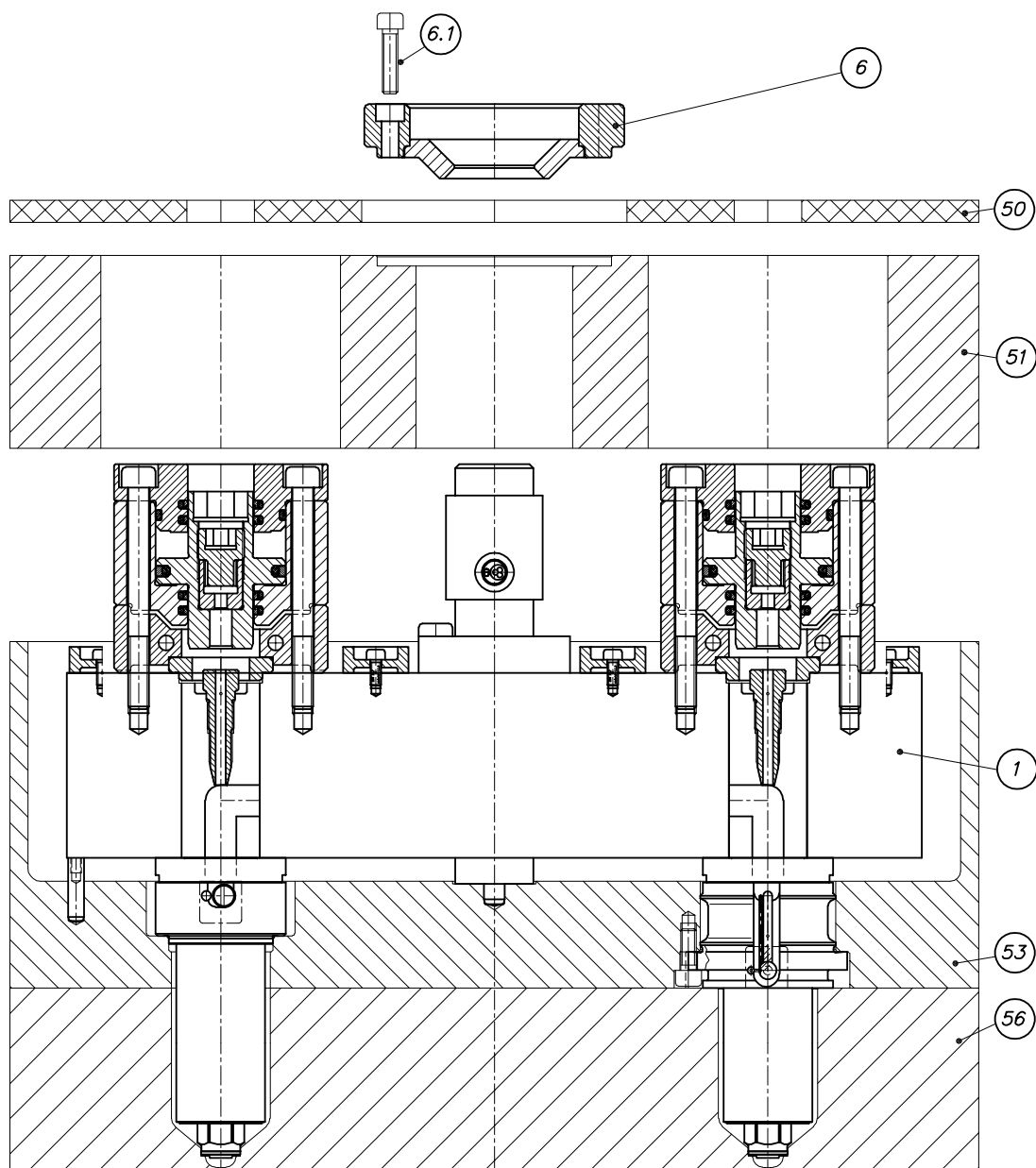
Abbildung 39: Montage der Aufspannplatte und des Zentrierrings
