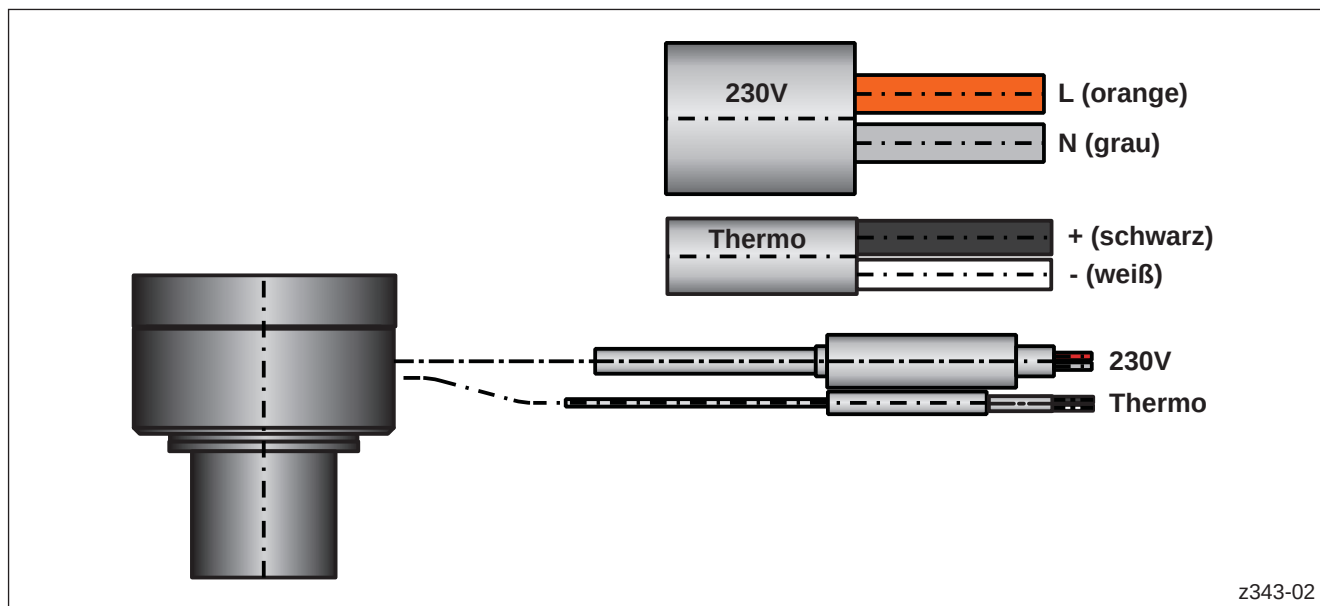
Abbildung 58: Kabelbelegung für HPS III-S Düsen (ein Regelkreis)
