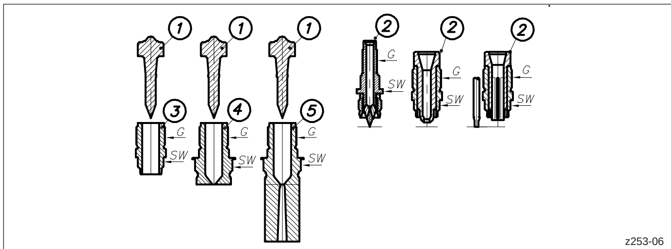
Abbildung 112: Beispiele von Düsenspitzen
