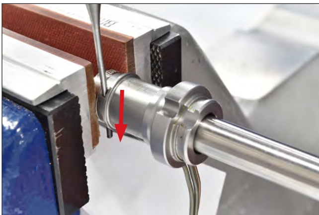
Abbildung 88: Spannhülse herausschlagen
