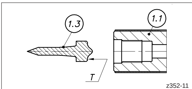
Abbildung 81: Düsenspitze herausziehen
