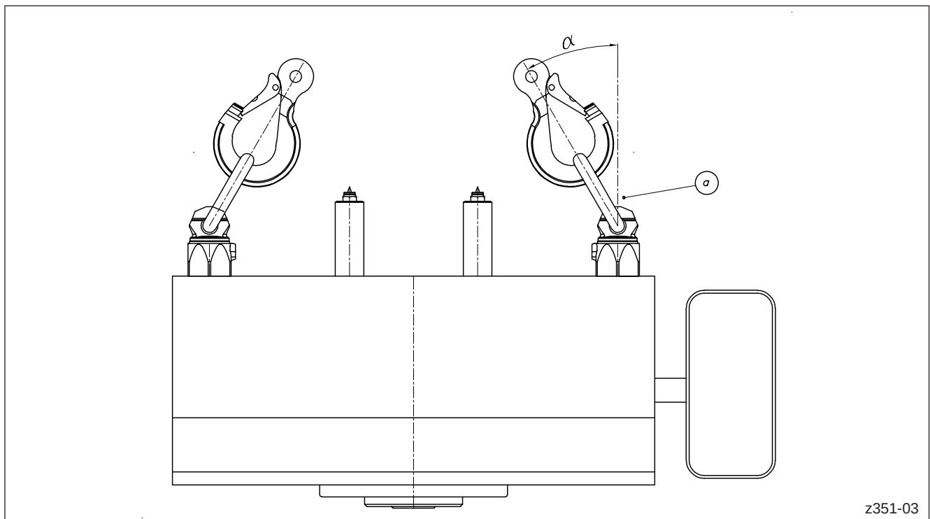
Abbildung 56: Vorbereitende Maßnahmen
