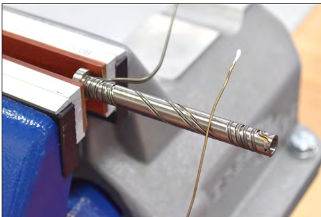
Abbildung 92: Benetzte Fühlerspitze
