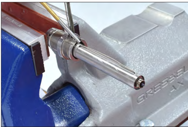
Abbildung 97: Klemmhülse abziehen
