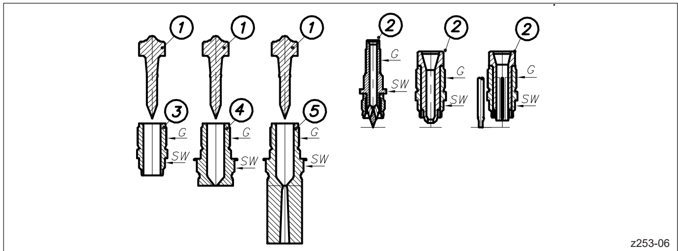
Abbildung 69: Beispiele von Düsenspitzen
