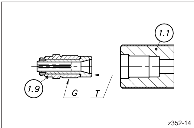
Abbildung 59: Düsenspitze montieren
