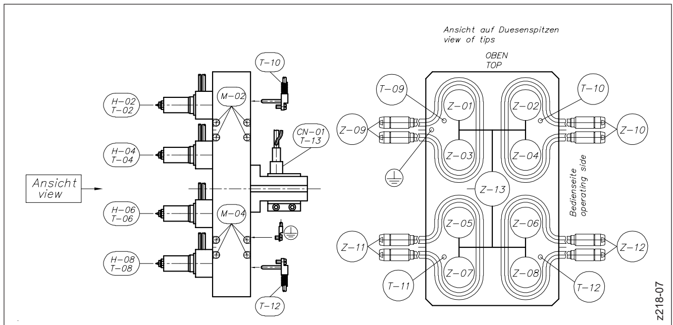
Abbildung 52: Verdrahtung von Standard-8-fach Heißkanalsystemen (Verteiler mit vier Regelkreisen)
