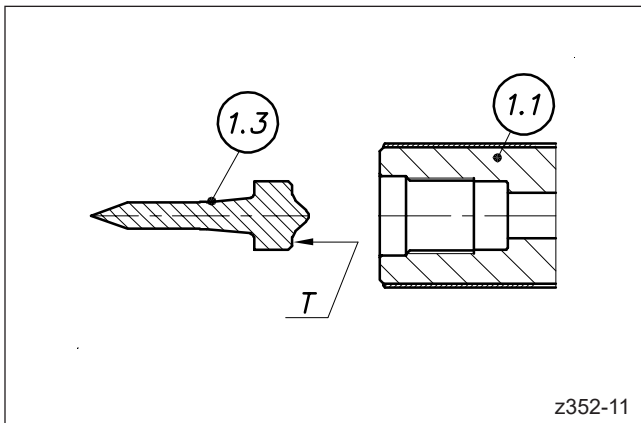
Abbildung 66: Düsenspitze montieren
