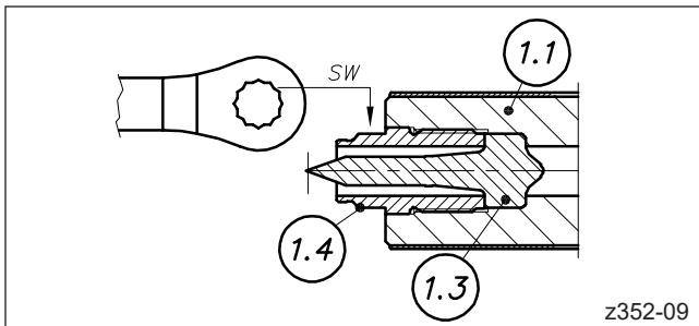
Abbildung 63: Mundstück herausschrauben
