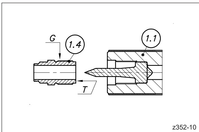
Abbildung 67: Düsenspitze montiert
