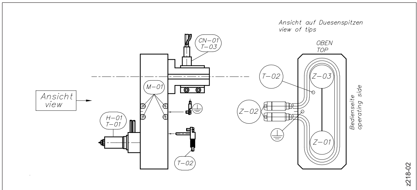
Abbildung 47: Verdrahtung von Standard-1-fach Heißkanalsystemen
